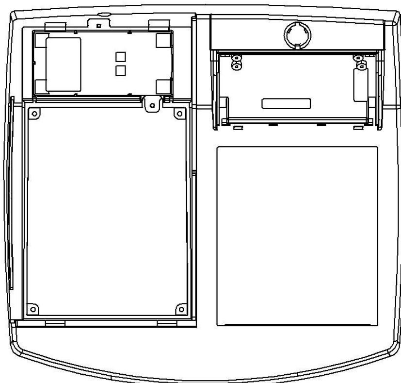
Рисунок 16 Корпус верхний ТКРП.0012.00.10.520
