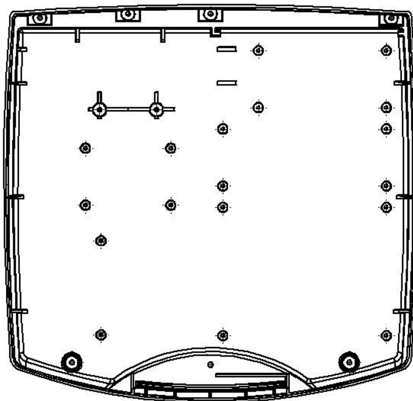
Рисунок 17 Корпус нижний ТКРП.0005.00.00.150
