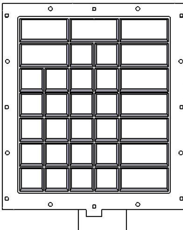
Рисунок 29 Блок клавиатуры ТКРП.0033.00.00.080
