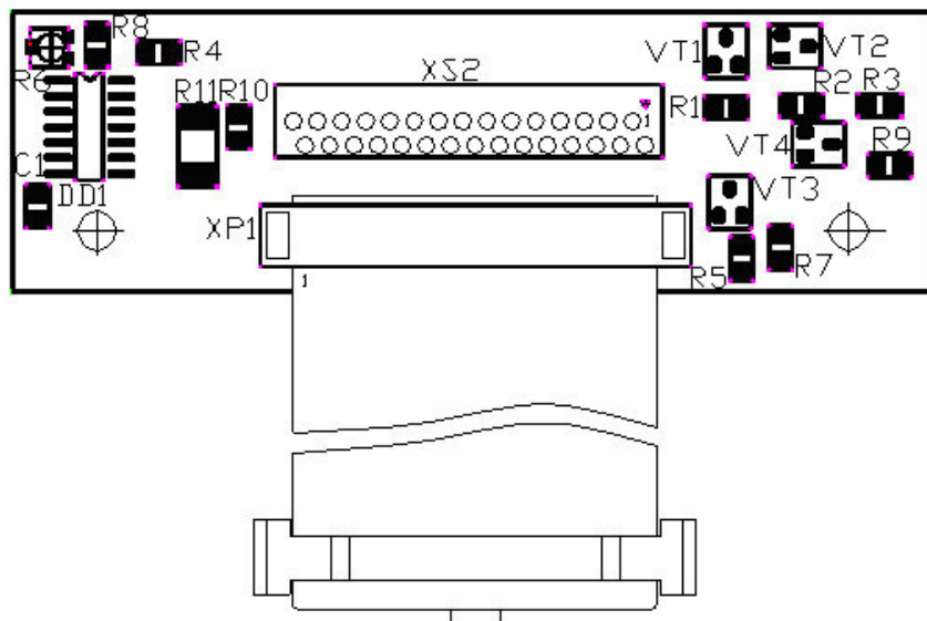
Рисунок 27 Переходной модуль ТКРП.0012.00.00.062
